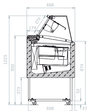
VETRO DRITTO / STRAIGHT GLASS GERADE SCHEIBE / VITRE DROITE
