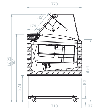
VETRO DRITTO / STRAIGHT GLASS GERADE SCHEIBE / VITRE DROITE
